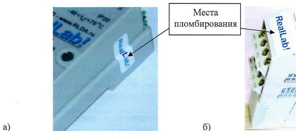
Рисунок 3 – Схема расположения мест пломбирования:
