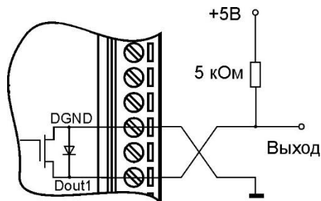
Рис. 6.8. Получения логических уровней напряжения на выходах модуля
