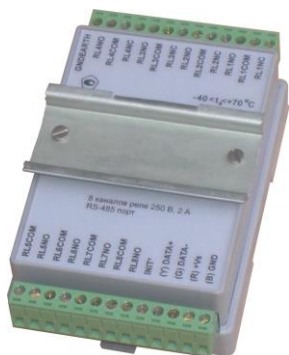
Рис. 6.3. Чтобы закрепить один модуль сверху другого, сначала закрепите DIN-рейку сверху модуля.
