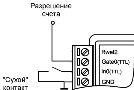
Рис. 6.5 . Подключение источника дискретных сигналов типа "сухой контакт" к модулю NL-2C-24V, взрывозащищённого исполнения
