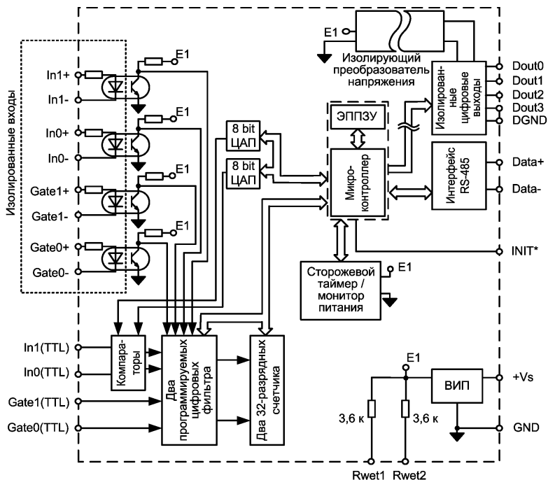
Рис. 4.1. Структурная схема модуля NL-2C-24V, взрывозащищённого исполнения
