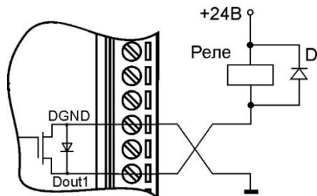
Рис. 6.7. Применение модуля для управления электромагнитным реле
