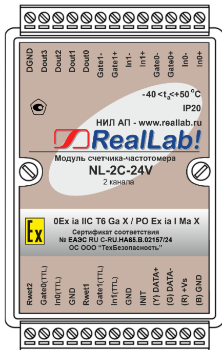
Рис. 2.1. Вид сверху на модуль NL-2C-24V, взрывозащищённого исполнения
