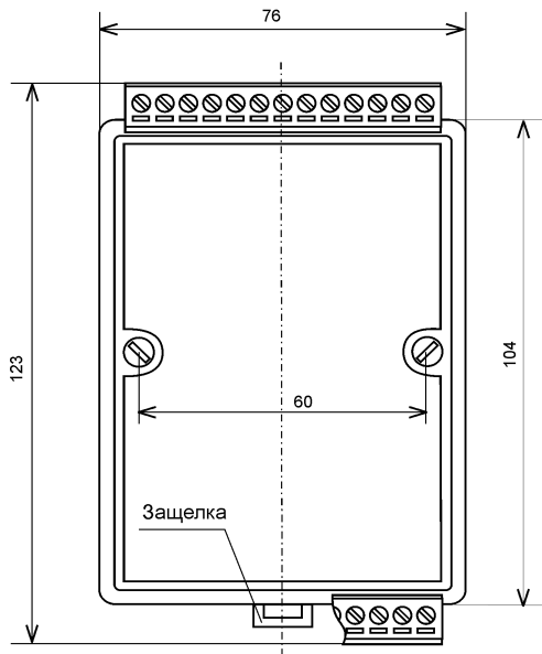
Рис. 2.2. Габаритный чертеж модуля
