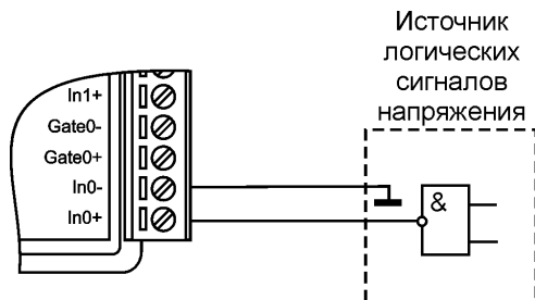
Рис. 6.9. Подключение источников логических сигналов к модулю. Счет разрешен программно
