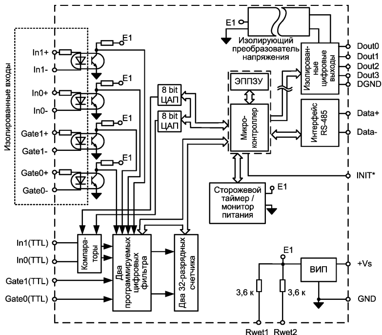
Рис. 4.1. Структурная схема модуля NL-2C-12V, взрывозащищенного исполнения
