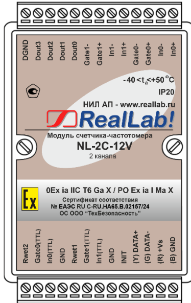
Рис. 2.1. Вид сверху на модуль NL-2C-12V, взрывозащищённого исполнения
